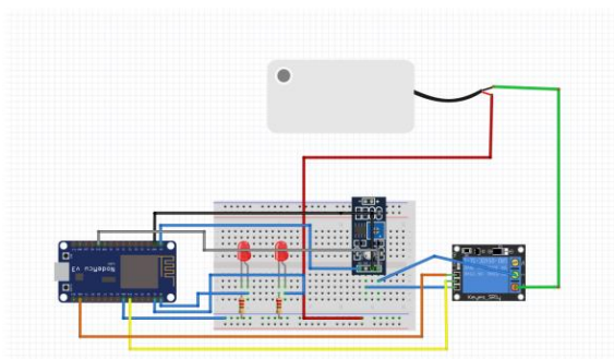
Gambar 2 Penyiraman tanaman otomatis fritzing
